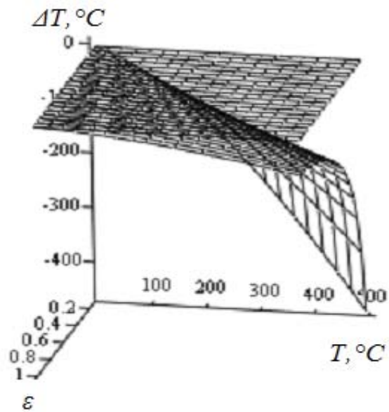
Рис. 2. Залежність методичної похибки вимірювання температури за випромінюванням від значення температури та коефіцієнта випромінювання, T_{\Phi} = 20 \text{ }^{\circ}\text{C}
