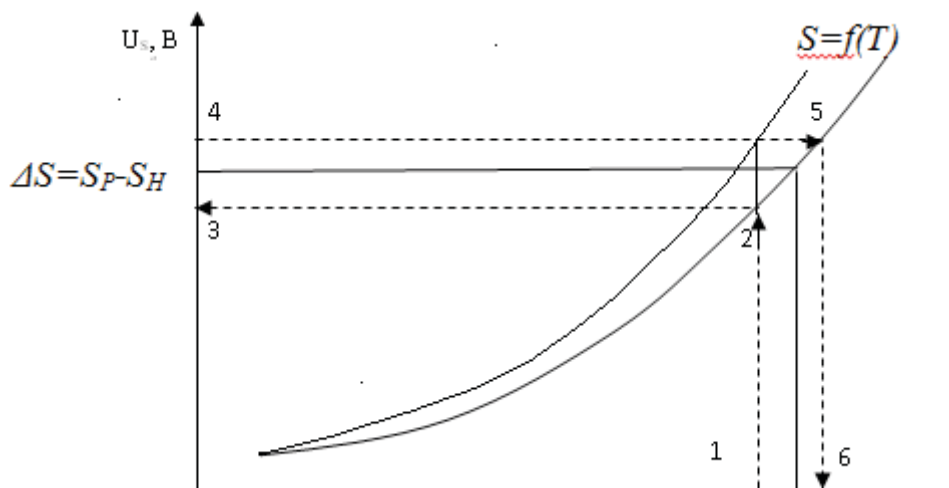
Рис. 1. Дія впливних факторів у робочих умовах виробництва на значення вимірюваної температури, яке визначається за калібрувальною функцією, встановленою в нормальних умовах
