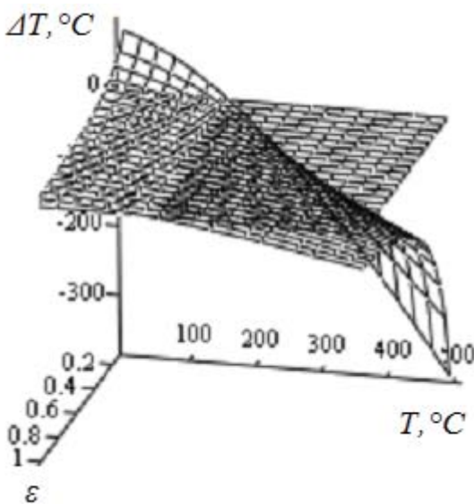
Рис. 3. Залежність методичної похибки вимірювання температури за випромінюванням від значення температури та коефіцієнта випромінювання, T_{\Phi} = 200 \text{ }^{\circ}\text{C}
