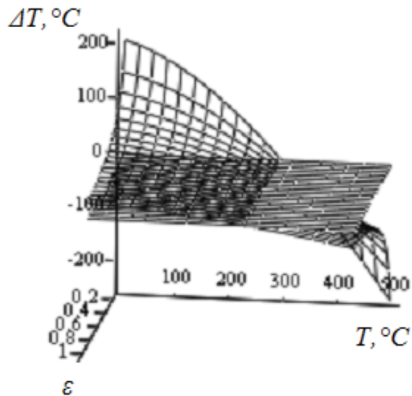
Рис. 4. Залежність методичної похибки вимірювання температури за випромінюванням від значення температури та коефіцієнта випромінювання, T_{\Phi} = 350 \text{ }^{\circ}\text{C}
