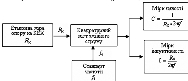
Рис. 10. Схема калібрування мір ємності та індуктивності за КЕХ
