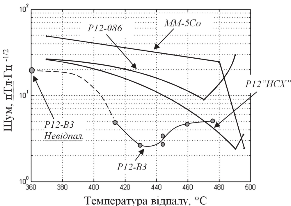
Рис. 2. Залежність рівня шумів від температури відпалу для різних модифікацій аморфного магнітного матеріалу \text{Co}_{88}\text{Fe}_3\text{Cr}_3\text{Si}_{15}\text{B}_{12}
